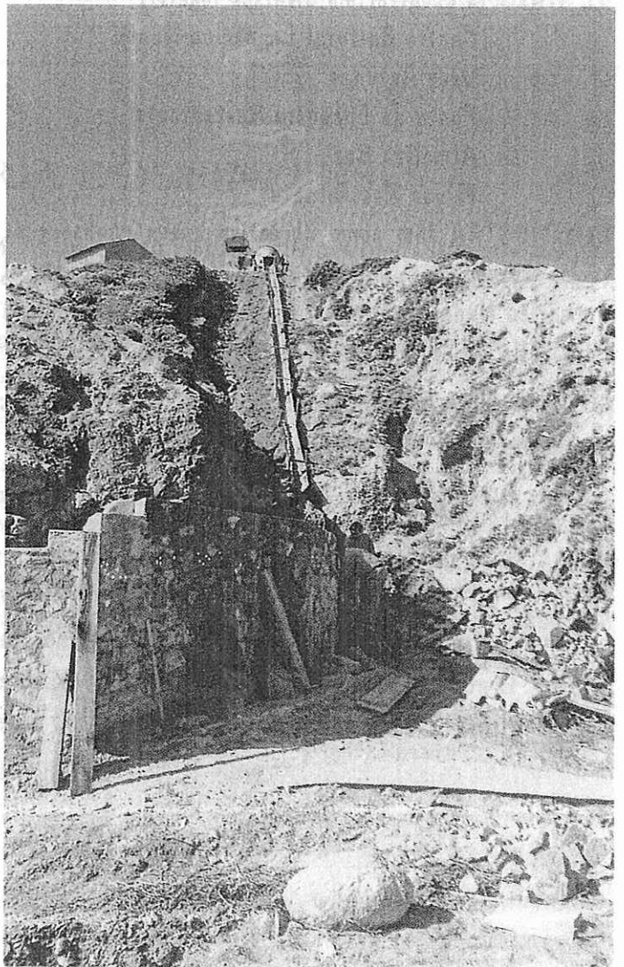
OBRAS DE ACESSO AO CANTO DO MOSQUEIRO
